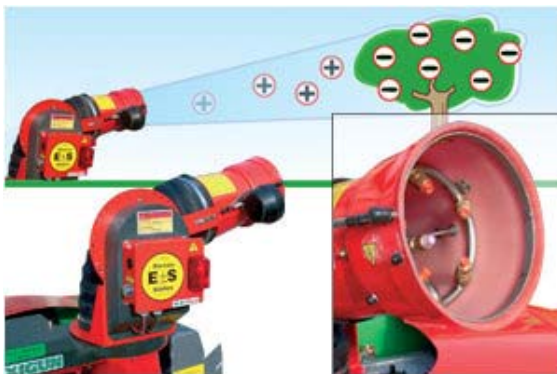
雾滴电荷充电系统
